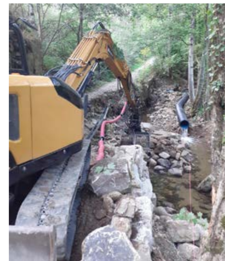
Mise en place des enrochements
